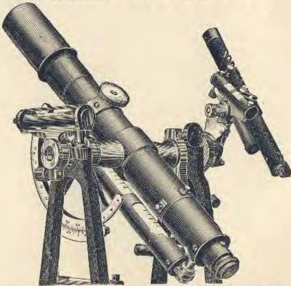
Buff & Berger's Latitude Level Attachment.
