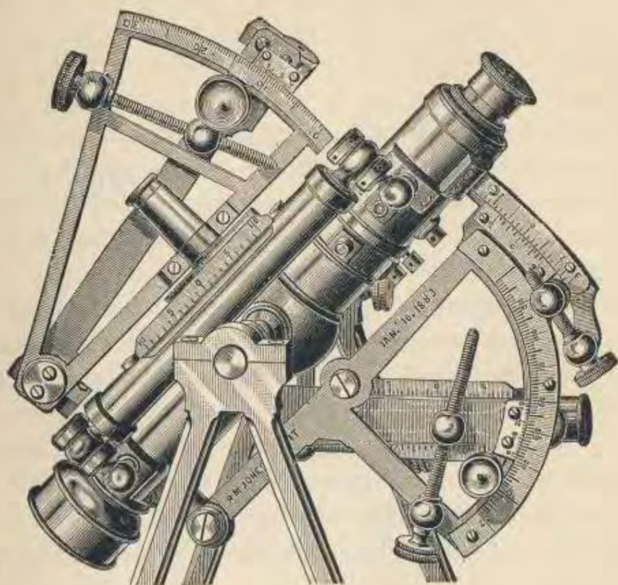
R. M. JONES' LATITUDE ARC.
