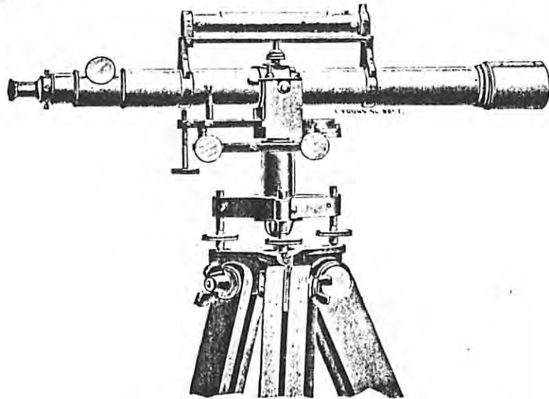
Wurdemann's Pivot Level.
