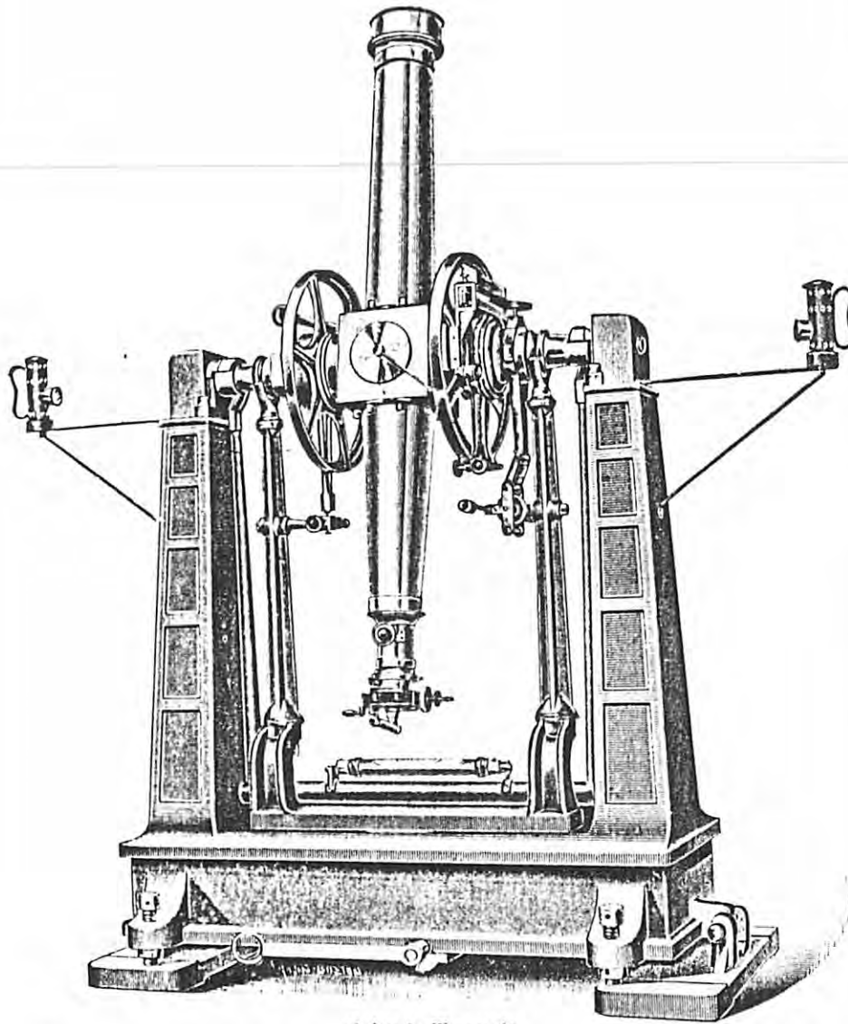
3-inch Transit.
