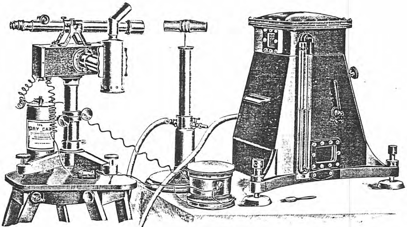
Coast Survey Pendulum Apparatus.
