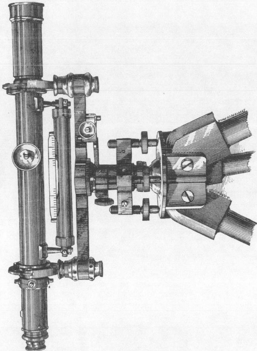
18 Inch Level.—No. 1.
