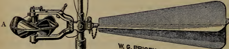
W. G. PRICE'S CURRENT-METER. W. & L. E. GURLEY. (Patented.)
